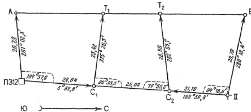
Разбивочный чертеж
