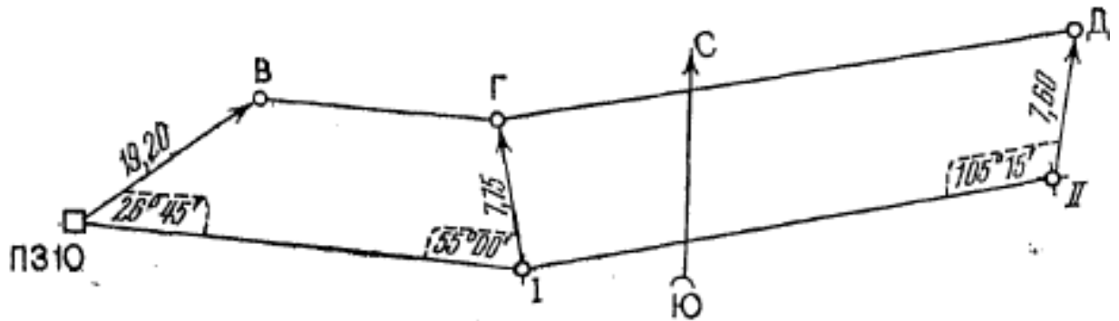
Разбивочный чертеж
